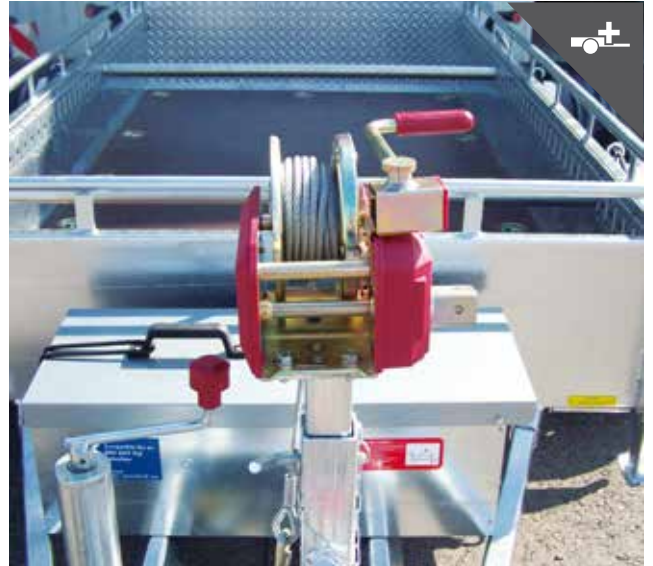
Handseilwinde auf Windenbock montiert
