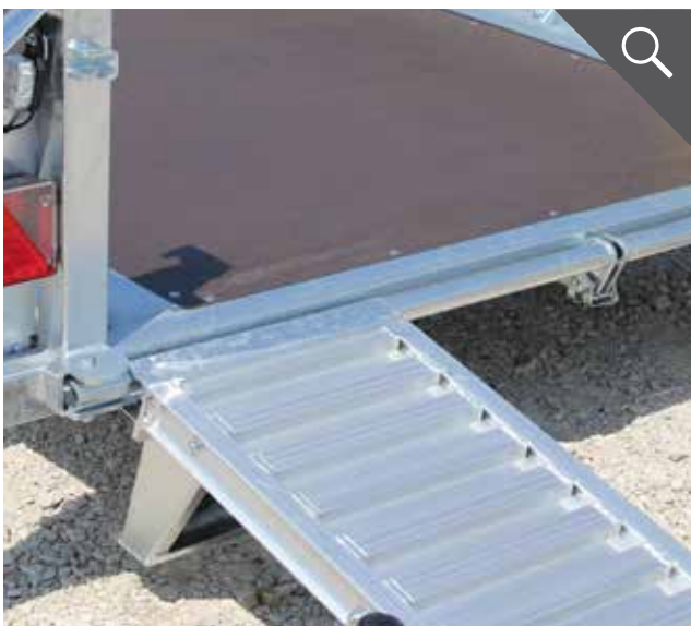
Auffahrrampen leicht zu verschieben für unterschiedliche Fahrzeugbreiten
